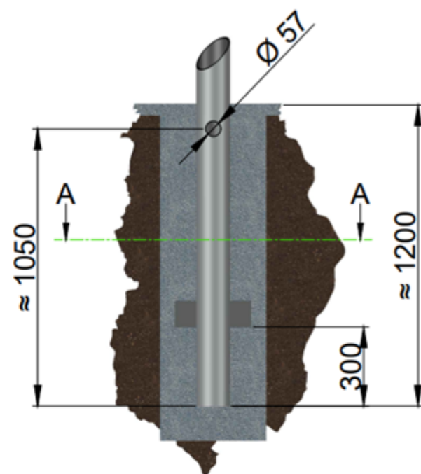
Detalhe engaste
