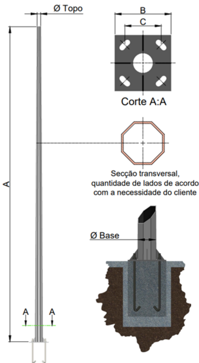
Poste conico continuo poligonal flangeado- DP-800
